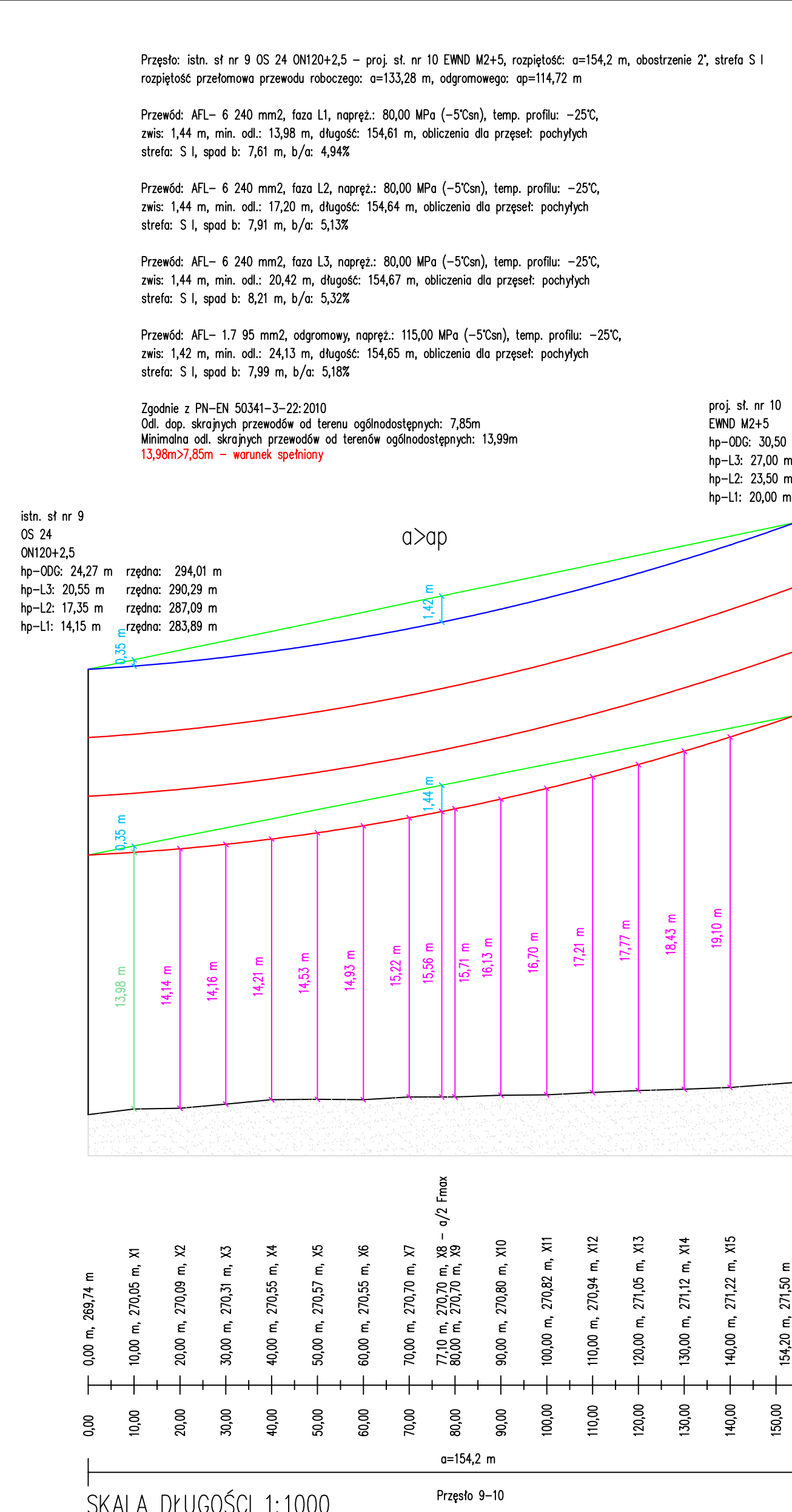
SKALA DŁUGOŚCI 1:1000
